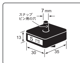
XV-02等のホルダーでは上図のピン向きで取り付けてください。
