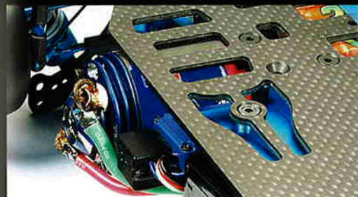
ロワデッキにはエアインテークとアルミ製エアダクトを装備
